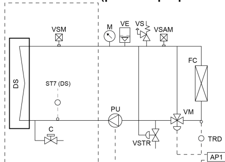
Installation à circuit ouvert (par exemple pour l'eau chaude sanitaire)
