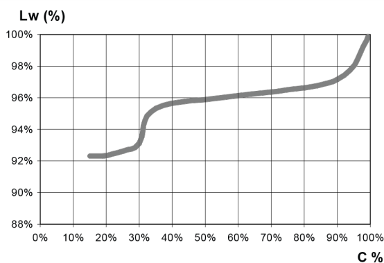
Graphique 1 - Niveau sonore Lw dB(A)
