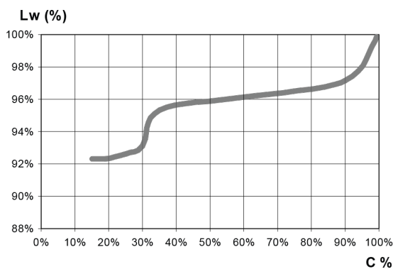
Gráfico 1 - Nivel sonoro Lw dB(A)
