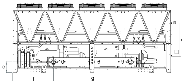
Detailansicht mit Pumpeinheit (Zubehör P/DP)
