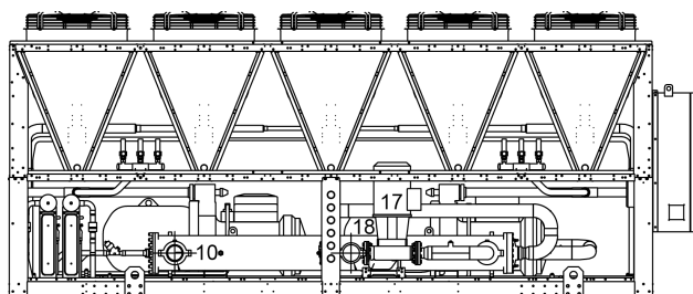
Detailansicht mit Pumpeinheit (Zubehör P/DP)
