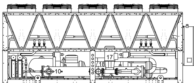
Vue détaillée avec kit hydraulique (accessoire P/DP)
